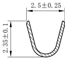
剖面 A-A
