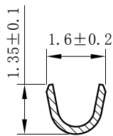
剖面 B-B
