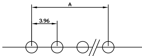
PCB 寸法
